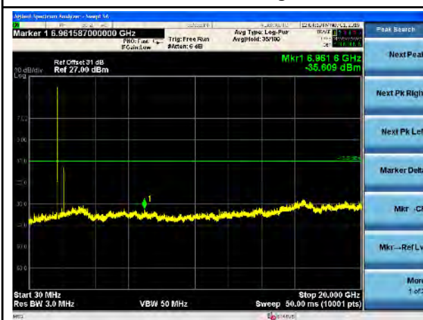
LTE Band 4, 10MHz-Mid CH
