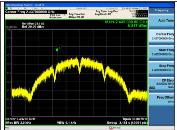
PSD-802.11b-Mid CH
