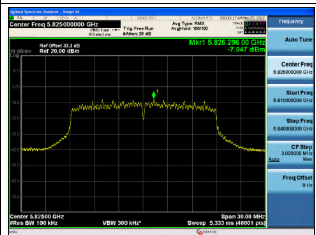
PSD_U-NII-3_802.11n_5825
