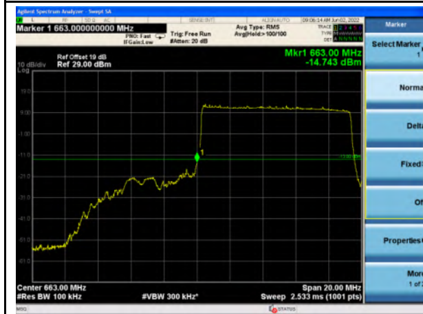
n71_10MHz_Lower Band Edge
