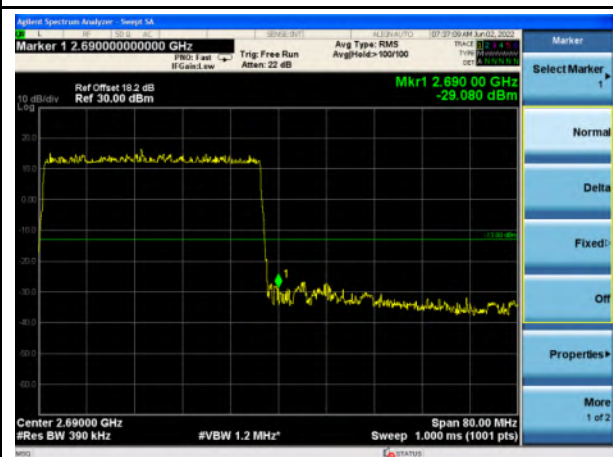
n41_40MHz_Upper Band Edge
