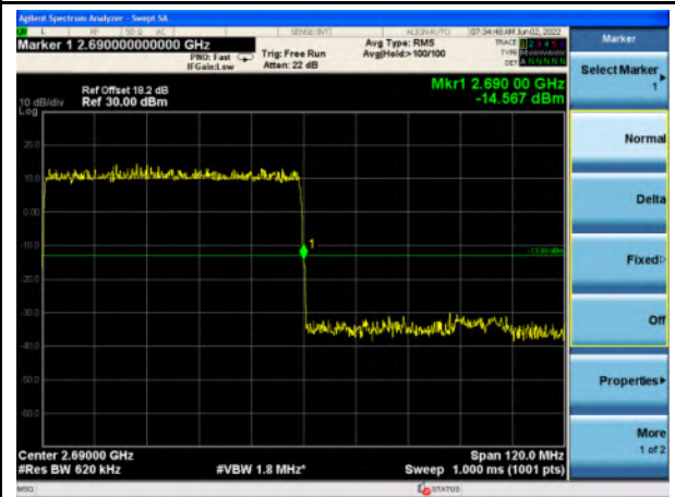
n41_60MHz_Upper Band Edge
