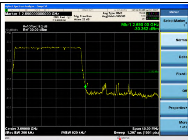
n41_20MHz_Upper Band Edge
