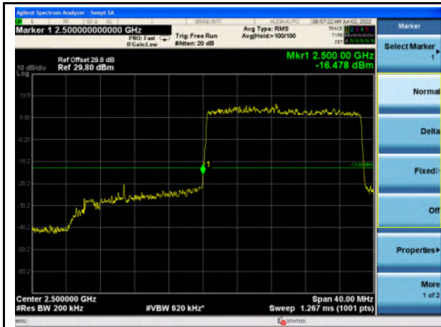
n7_20MHz_Lower Band Edge
