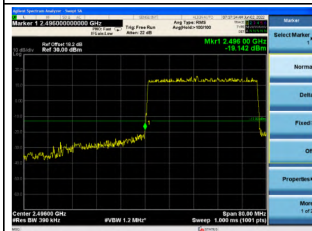
n41_40MHz_Lower Band Edge
