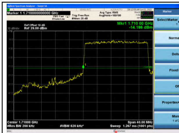
n66_20MHz_Lower Band Edge
