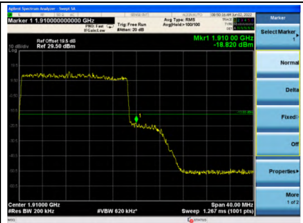
n2_20MHz_Upper Band Edge
