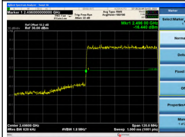
n41_60MHz_Lower Band Edge
