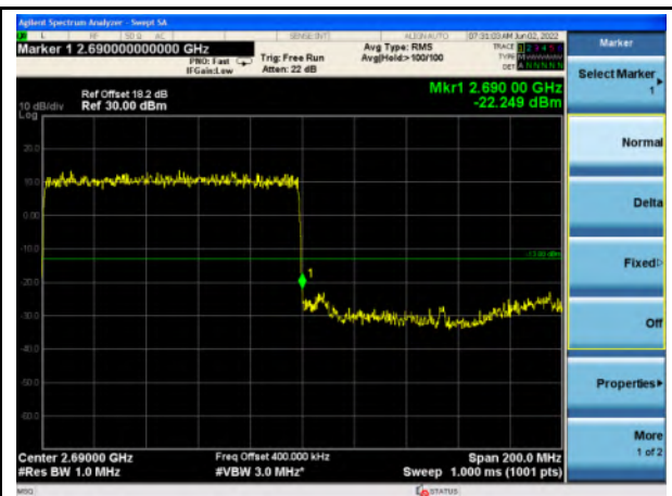
n41_100MHz_Upper Band Edge
