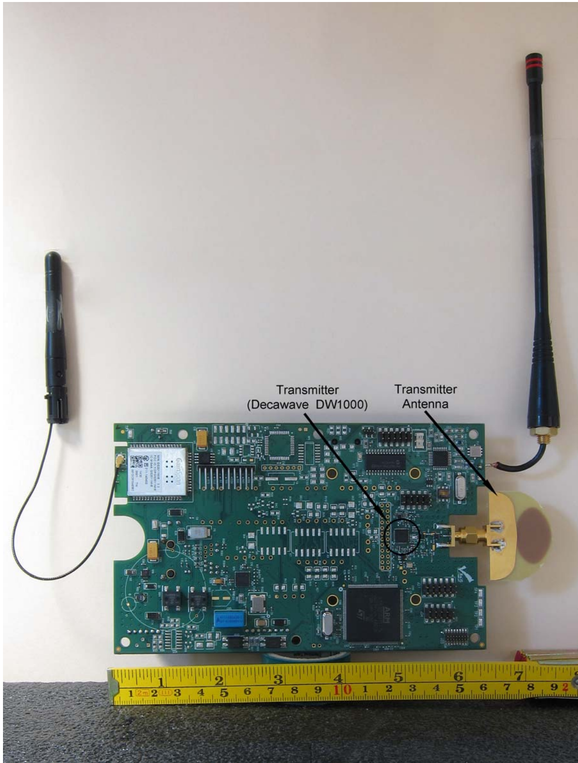
Module Rear
