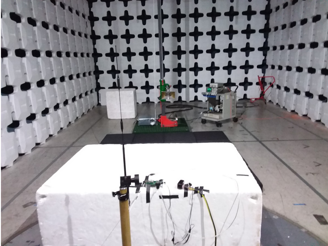
5dBi Omni
