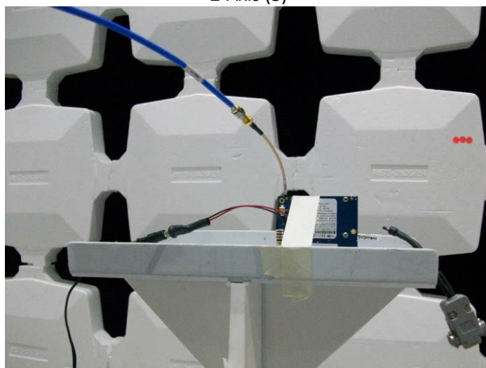
Z-Axis (3)
