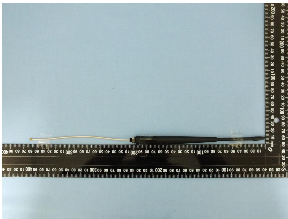
Antenna model: 0600-00048
