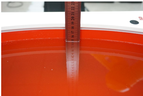
HSL_2300MHz-2700MHz_15.1cm
