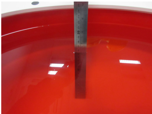
HSL_1900MHz-2300MHz_15.4cm
