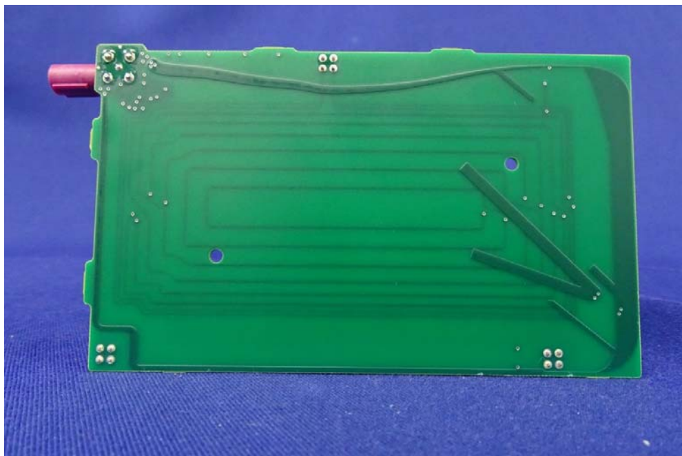
(9) EUT Photo
