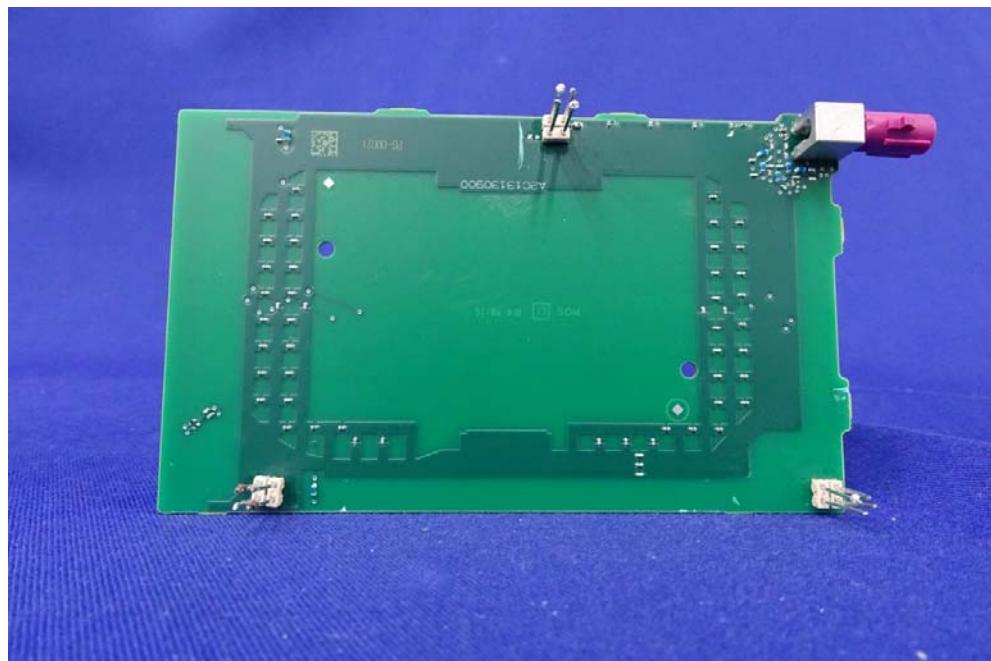
(8) EUT Photo
