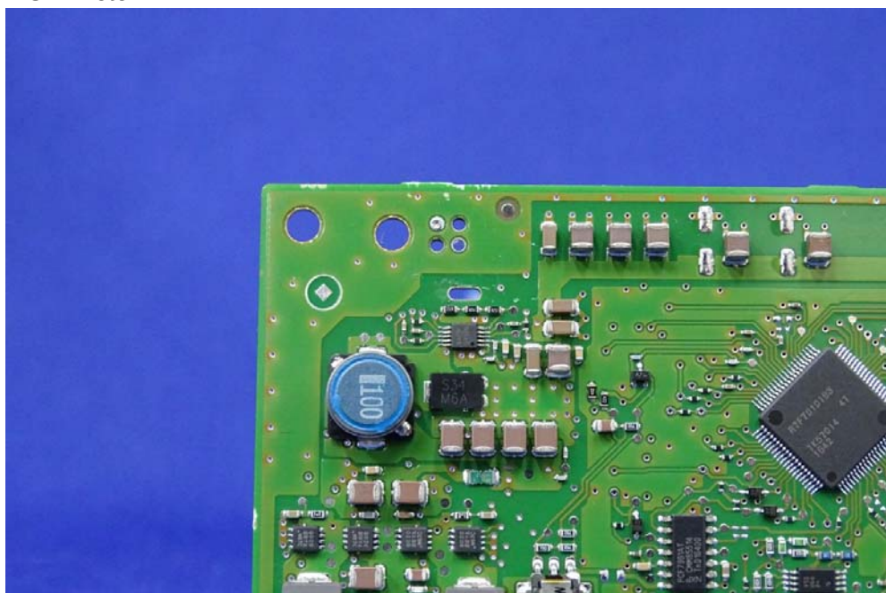
(14) EUT Photo
