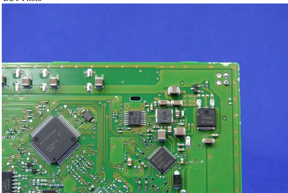
(16) EUT Photo
