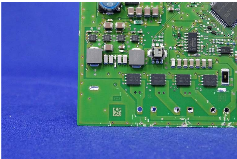
(15) EUT Photo
