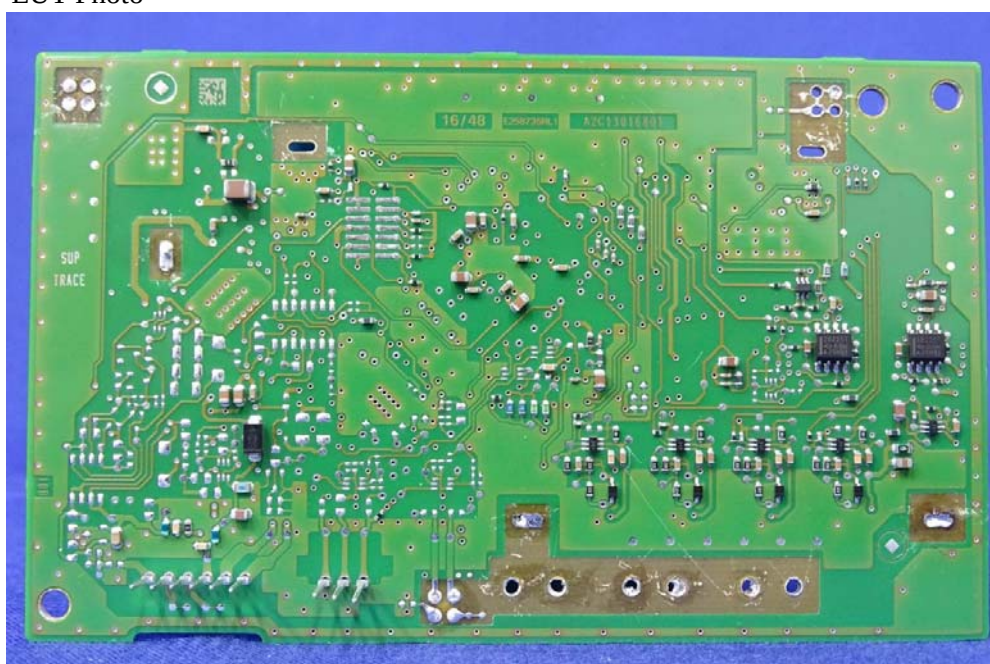
(10) EUT Photo
