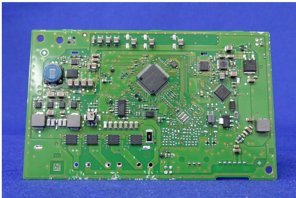
(13) EUT Photo
