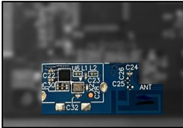
Bluetooth IC & PCB Antenna
