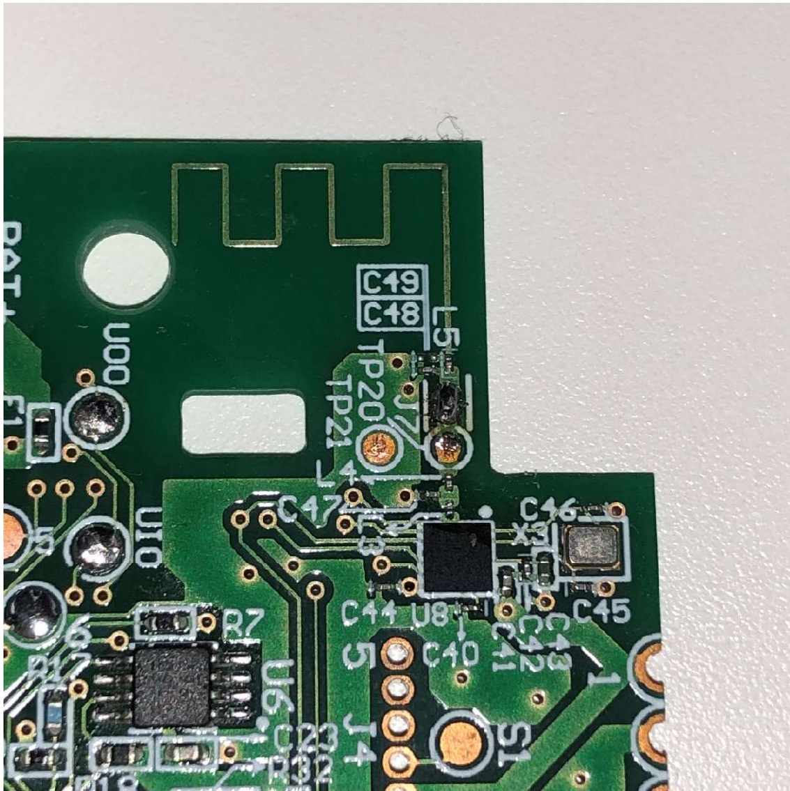
BLE IC & Antenna
