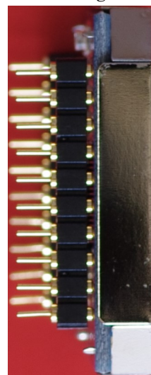
右側面 Right side
