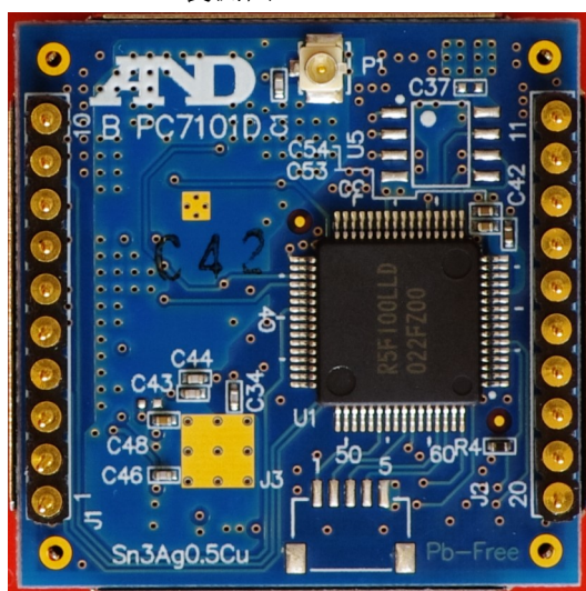
裏側面 Back side
