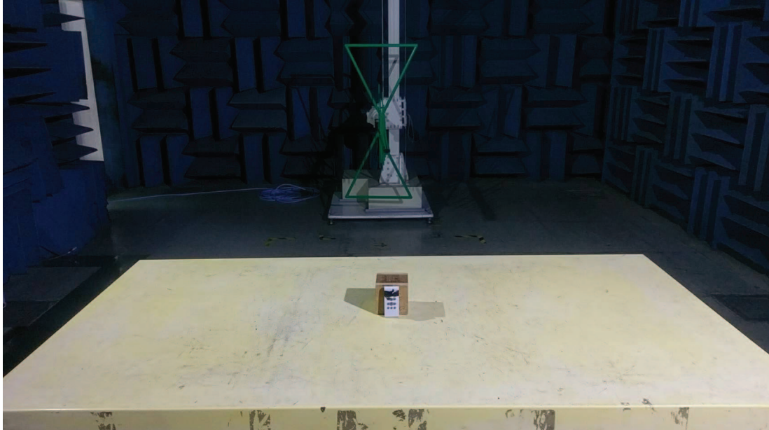
EUT on Stand
