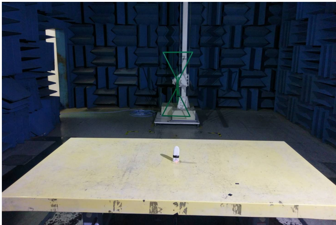
EUT on Stand
