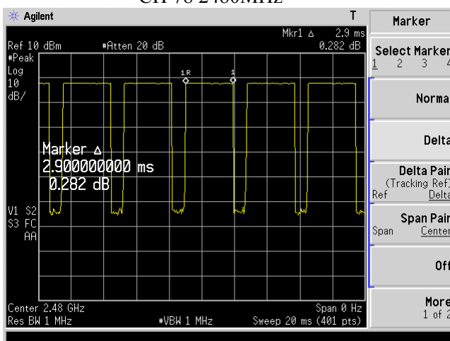
CH 78 2480MHz
