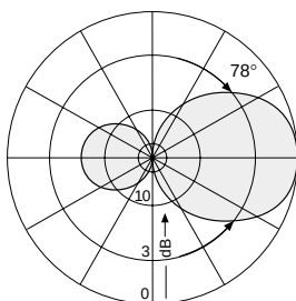
Vertikal 60 mm Ø
