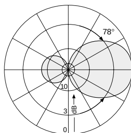
Vertikal 115 mm Ø
