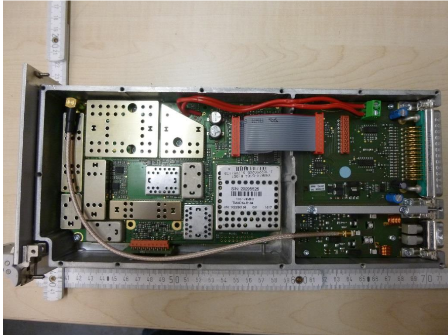
Photo 41: RF module
