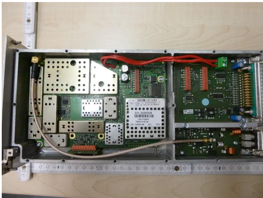
Photo 42: RF module
