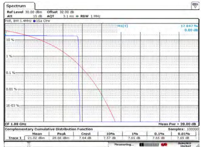
Figure 1-30a: PCS1900 Band, PAR Mid Channel
