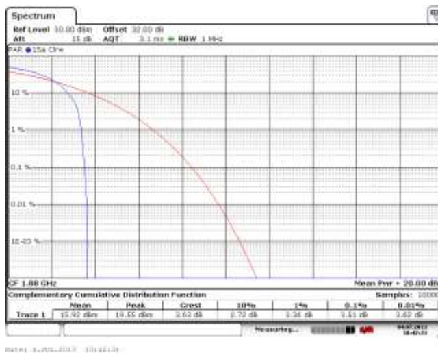
Figure 2-30a: Band 2, PAR Mid Channel
