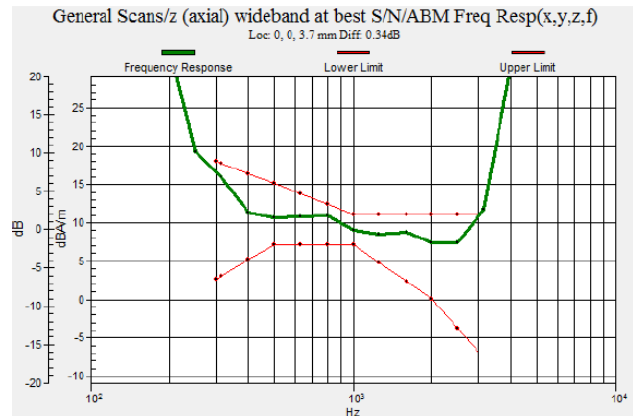
Fig 7.2 GSM850 Ch189
