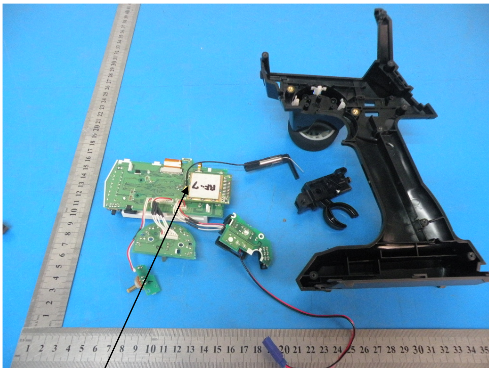
Antenna
