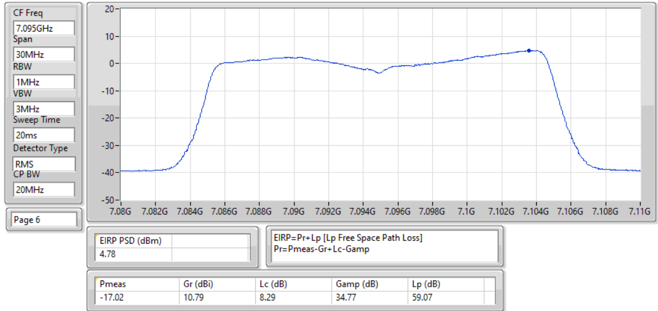
EIRP PSD;Band:7.0G;ax20,BF;BWch:20MHz;Nss:1,(M0);Nant:2;Ch:7095MHz;TX
