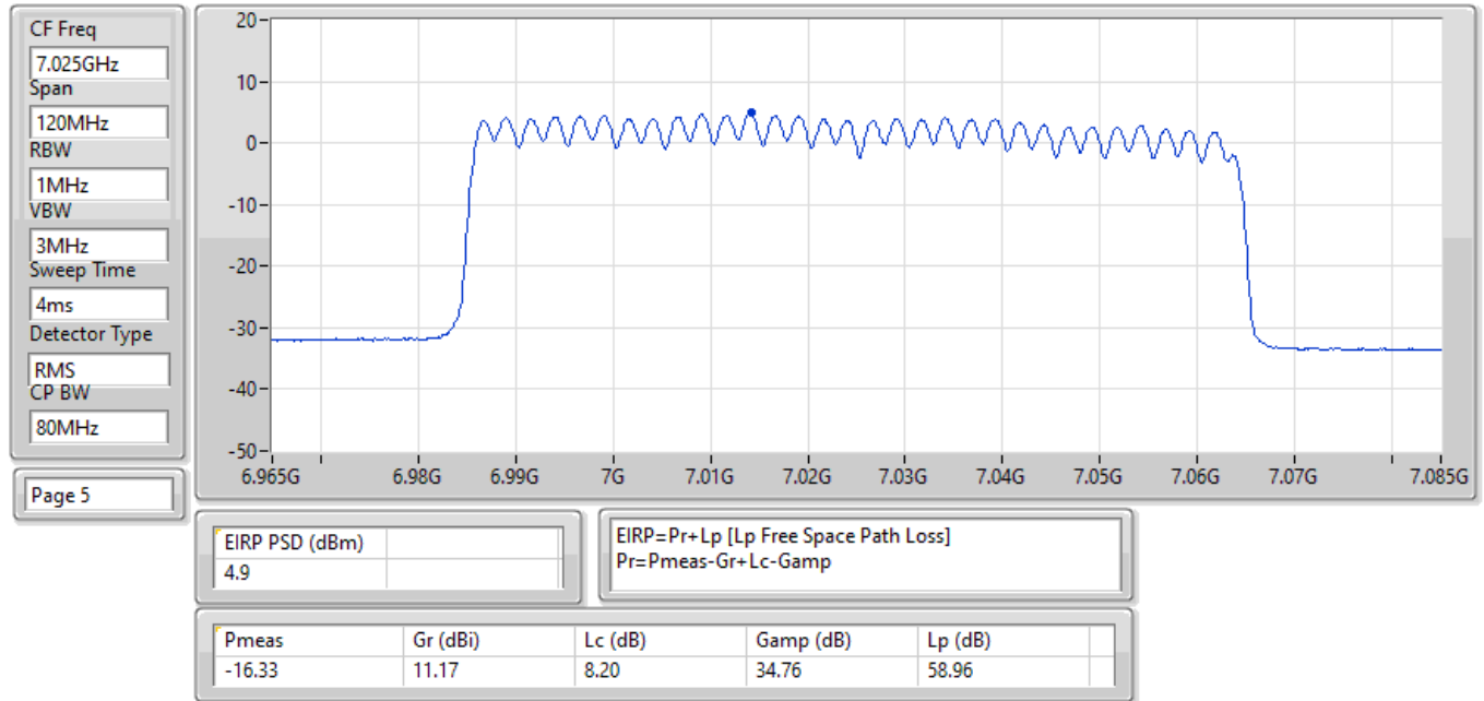
EIRP PSD;Band:7.0G;ax80;BWch:80MHz;Nss:1,(M0);Nant:2;Ch:7025MHz;TX
