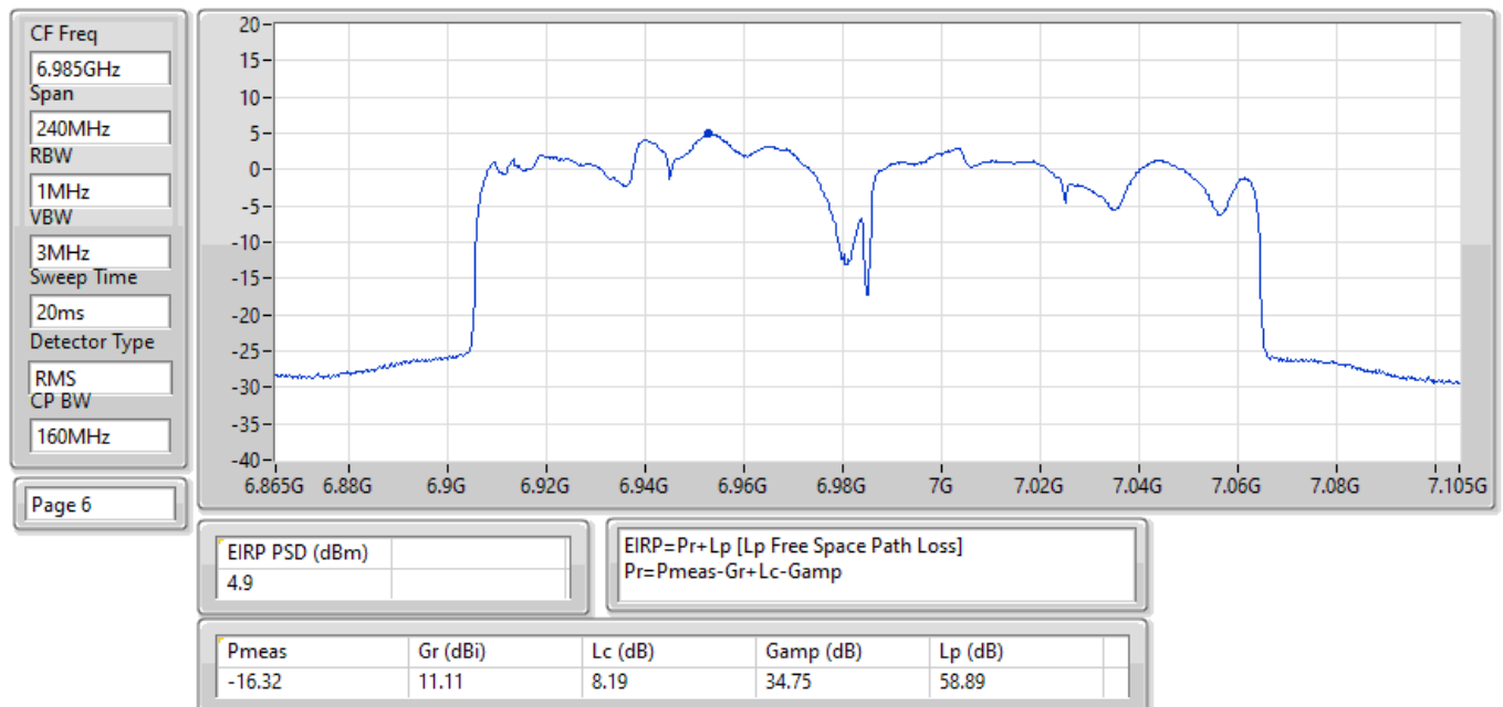
EIRP PSD;Band:7.0G;ax160,BF;BWch:160MHz;Nss:1,(M0);Nant:2;Ch:6985MHz;TX
