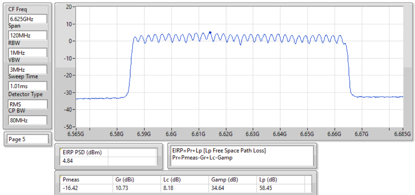
EIRP PSD;Band:6.7G;ax80;BWch:80MHz;Nss:1,(M0);Nant:2;Ch:6625MHz;TX
