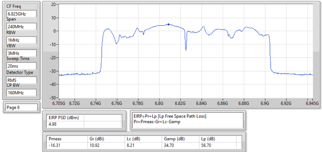
EIRP PSD;Band:6.7G;ax160,BF;BWch:160MHz;Nss:1,(M0);Nant:2;Ch:6825MHz;TX
