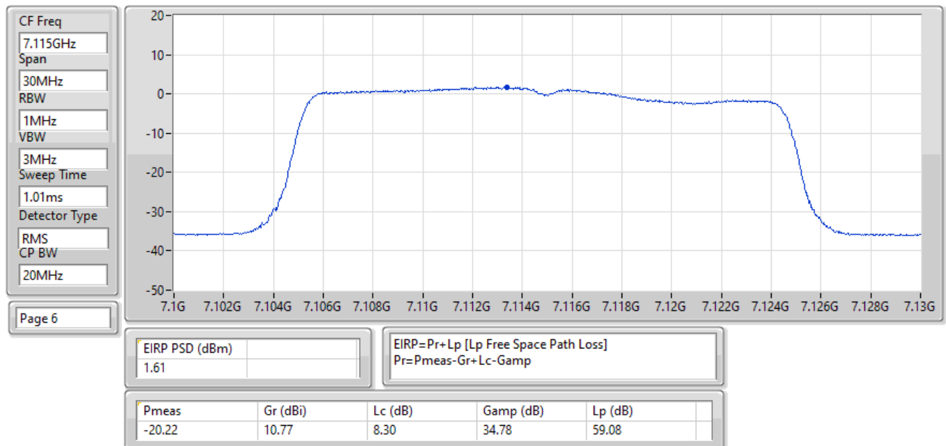
EIRP PSD;Band:7.0G;ax20,BF;BWch:20MHz;Nss:1,(M0);Nant:2;Ch:7115MHz;TX
