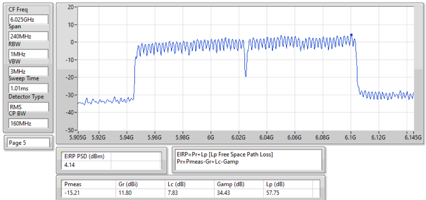
EIRP PSD;Band:6.2G;ax160;BWch:160MHz;Nss:1,(M0);Nant:2;Ch:6025MHz;TX
