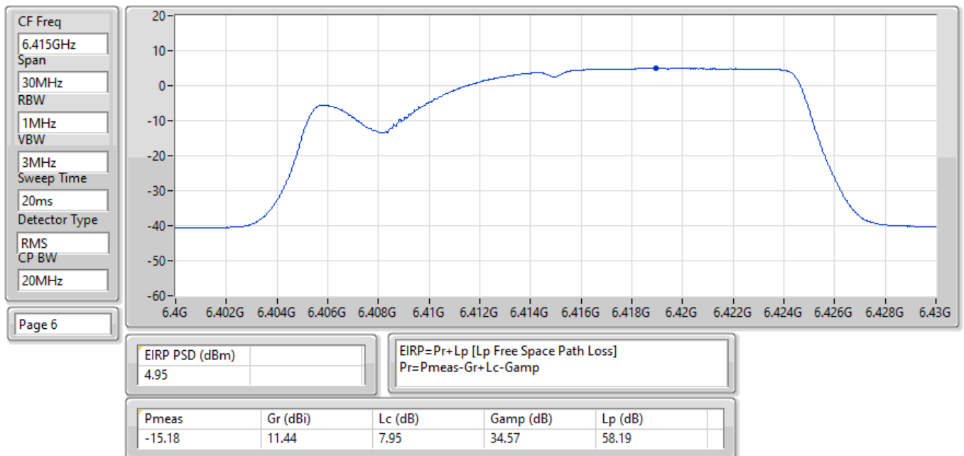
EIRP PSD;Band:6.2G;ax20,BF;BWch:20MHz;Nss:1,(M0);Nant:2;Ch:6415MHz;TX
