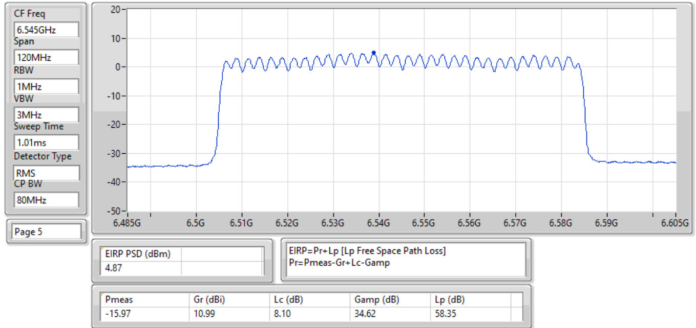
EIRP PSD;Band:6.4G;ax80;BWch:80MHz;Nss:1,(M0);Nant:2;Ch:6545MHz;TX
