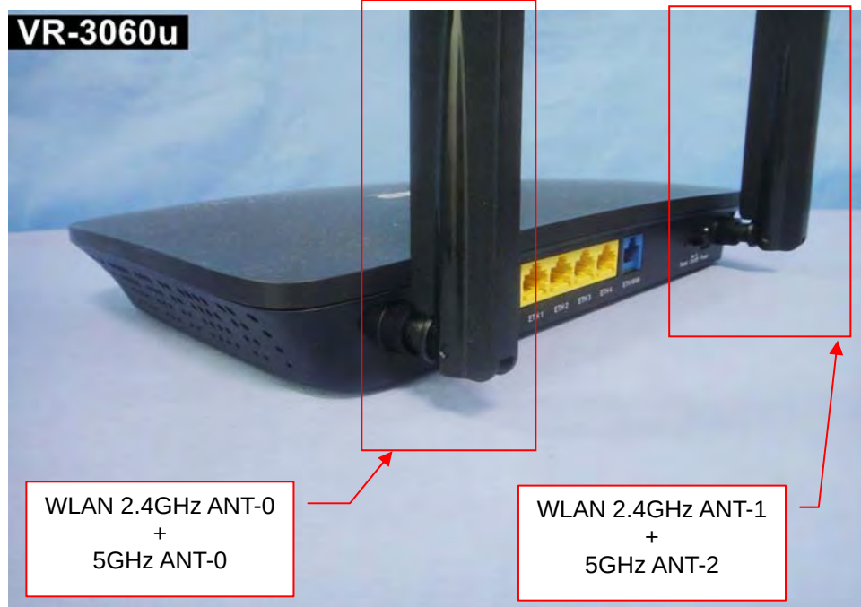
EUT Photo 3 )
