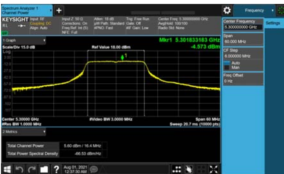
Antenna A
