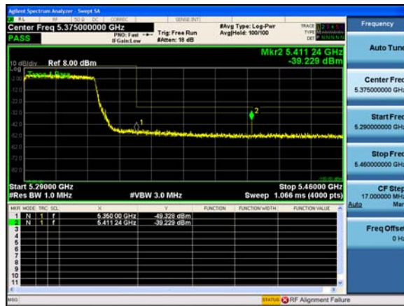
Antenna A
