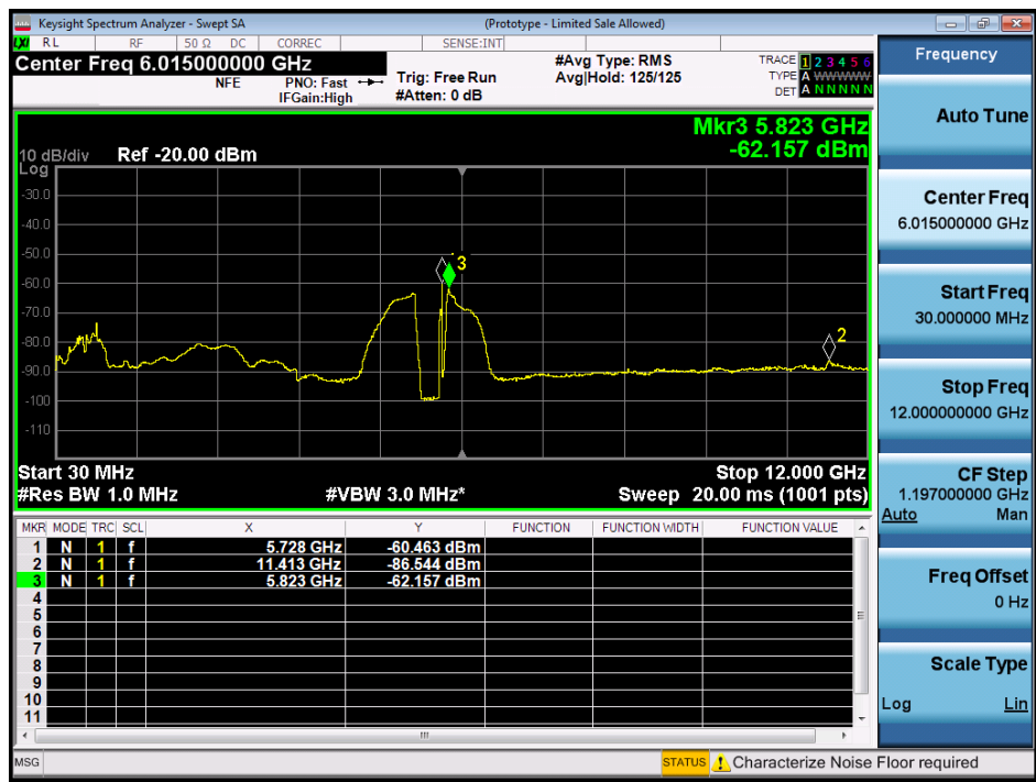
Antenna A
