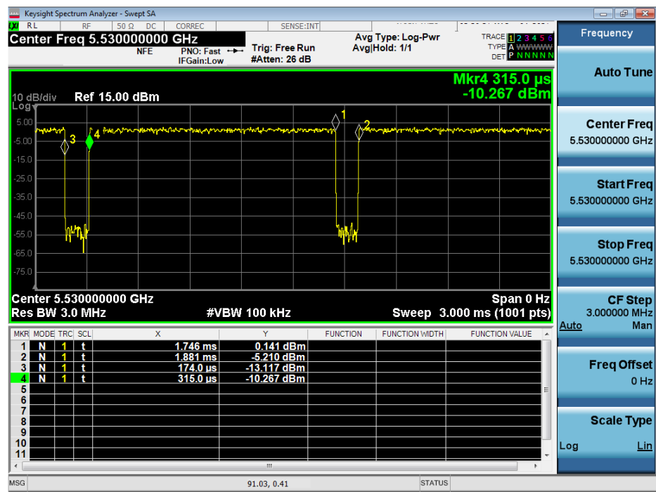
Antenna A
