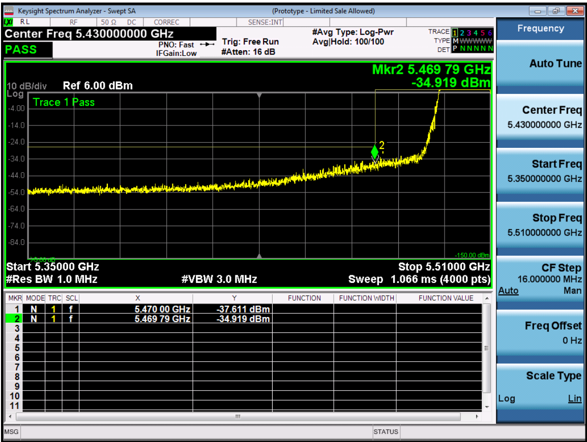
Antenna A
