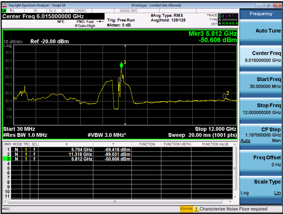
Antenna A
