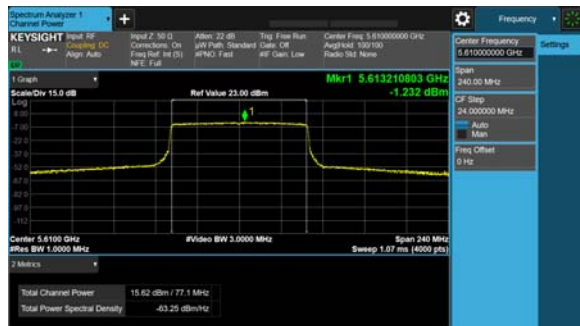
Antenna A
