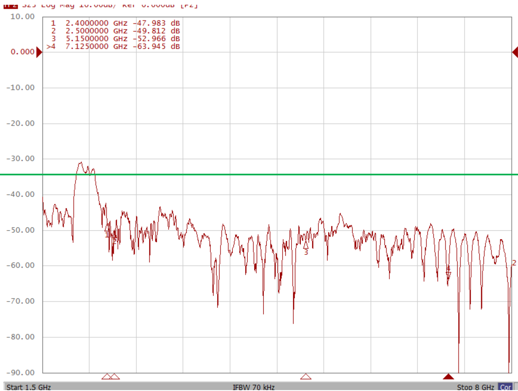
WIFI1 & BT
