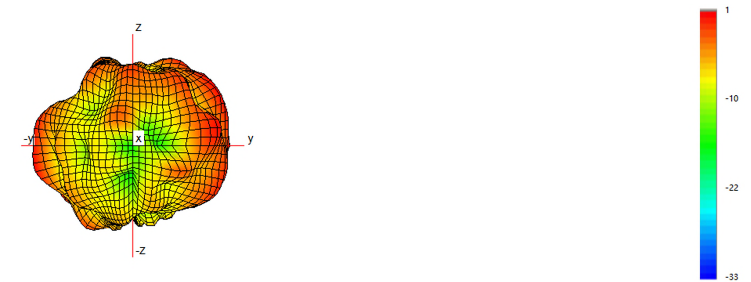
@6.5GHz
