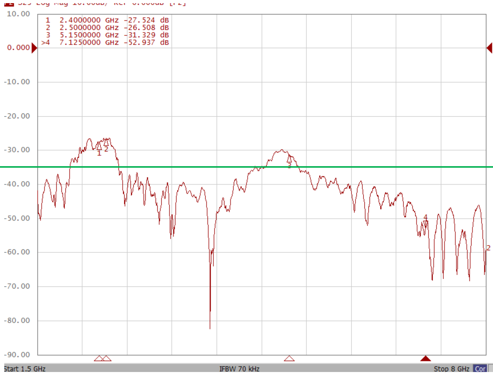
WIFI2 & BT
