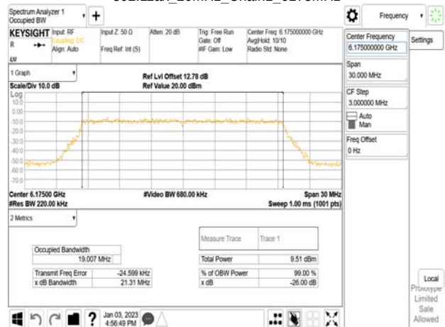
802.11ax_20MHz_Chain1_6175MHz
