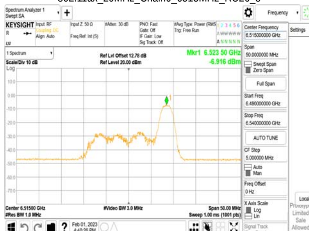
802.11ax_20MHz_Chain0_6515MHz_RU52_40
