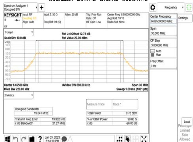
802.11ax_20MHz_Chain1_6695MHz
