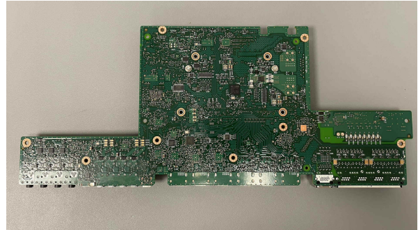
PCB bottom
