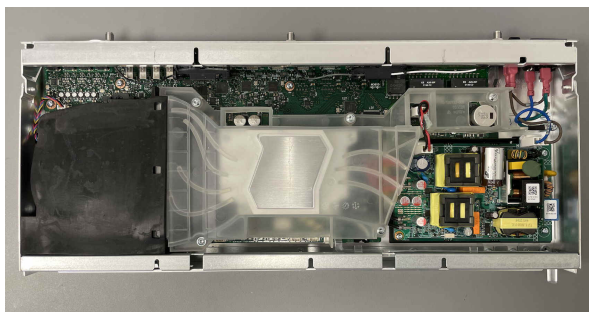
Incl. airguide
