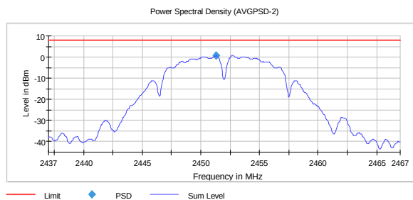
PSD, 2452 MHz, 802.11b 1M 0.7
