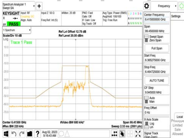
802.11ax_20MHz_Chain0_6415MHz_RU52_40
