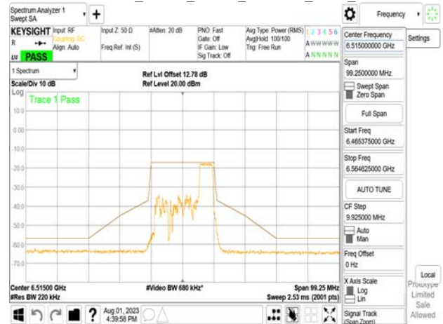
802.11ax_20MHz_Chain1_6515MHz_RU52_40
