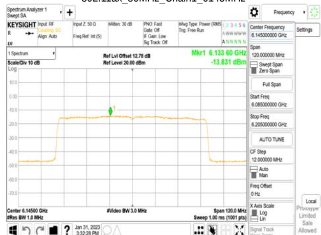
802.11ax_80MHz_Chain1_6145MHz
