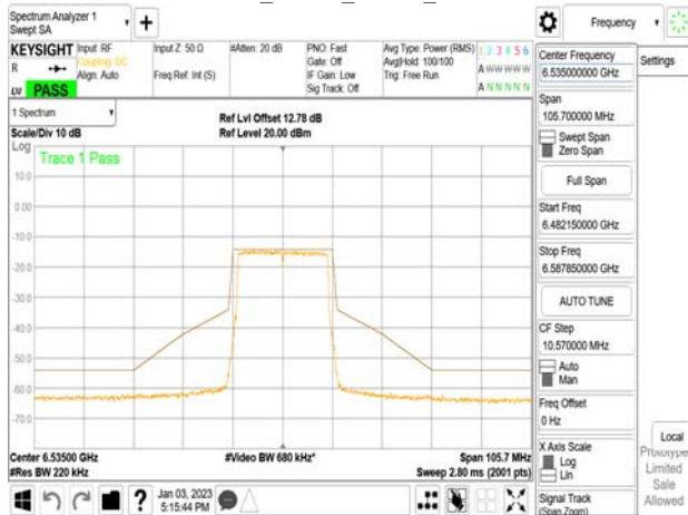
802.11ax_20MHz_Chain0_6535MHz_RU26_0
