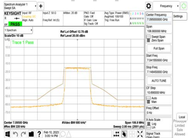
802.11ax_20MHz_Chain0_7095MHz_RU26_8
