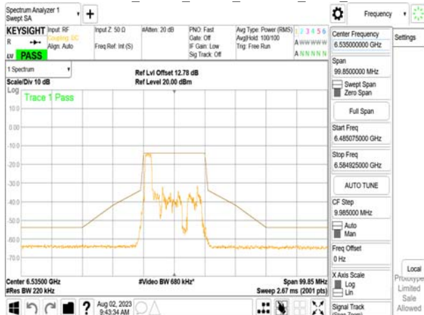
802.11ax_20MHz_Chain0_6535MHz_RU26_0
