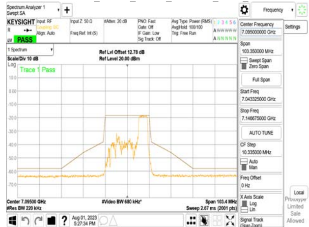
802.11ax_20MHz_Chain0_7095MHz_RU52_40
