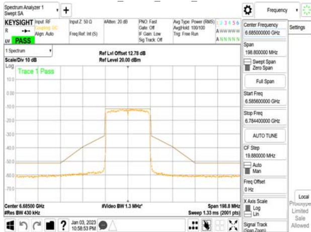
802.11ax_40MHz_Chain0_6685MHz
