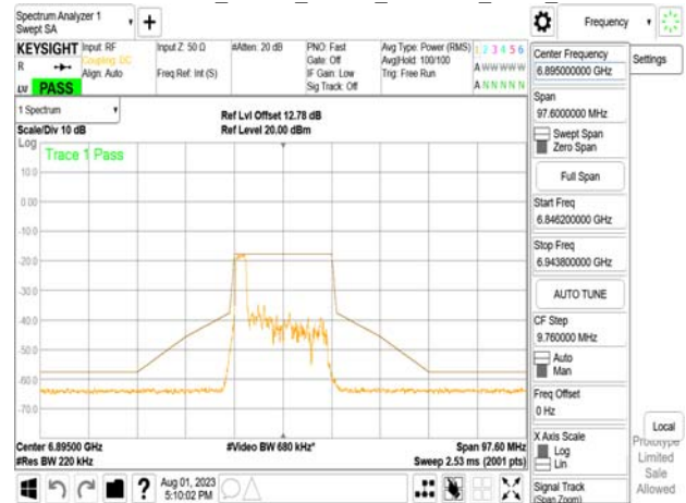
802.11ax_20MHz_Chain0_6895MHz_RU26_0
