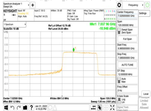
802.11ax_80MHz_Chain1_7025MHz_RU484_66
