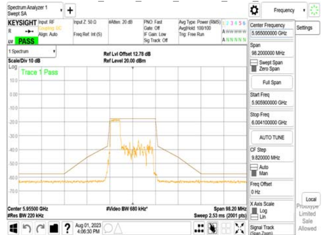
802.11ax_20MHz_Chain1_5955MHz_RU106_53
