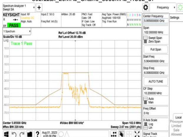
802.11ax_20MHz_Chain0_5955MHz_RU52_37
