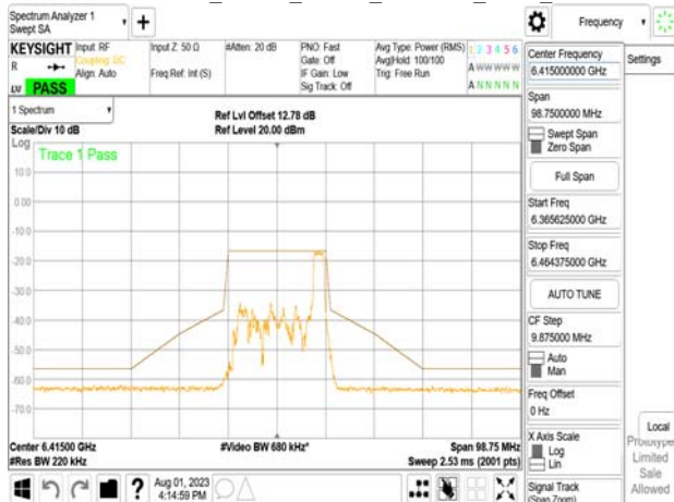
802.11ax_20MHz_Chain1_6415MHz_RU52_40
