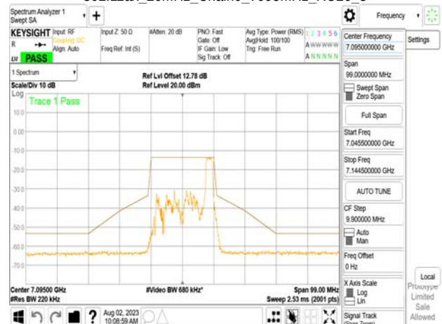
802.11ax_20MHz_Chain0_7095MHz_RU26_8
