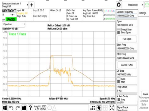
802.11ax_20MHz_Chain1_5955MHz_RU26_0
