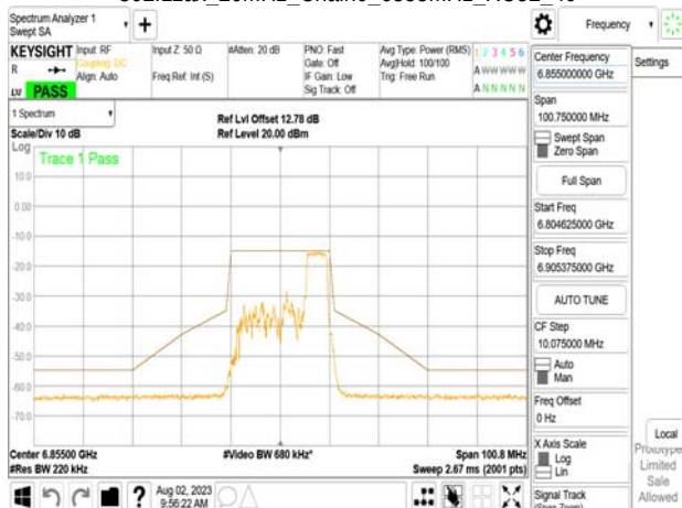
802.11ax_20MHz_Chain0_6855MHz_RU52_40
