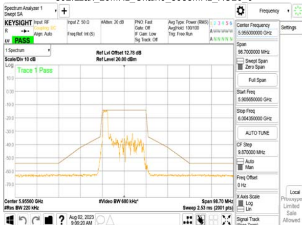
802.11ax_20MHz_Chain0_5955MHz_RU26_0
