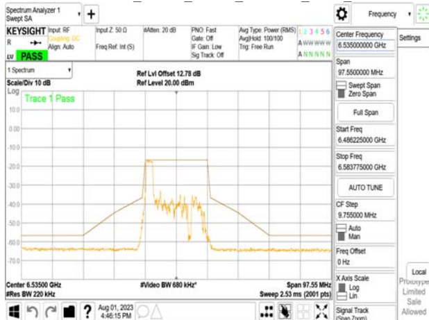
802.11ax_20MHz_Chain0_6535MHz_RU52_37
