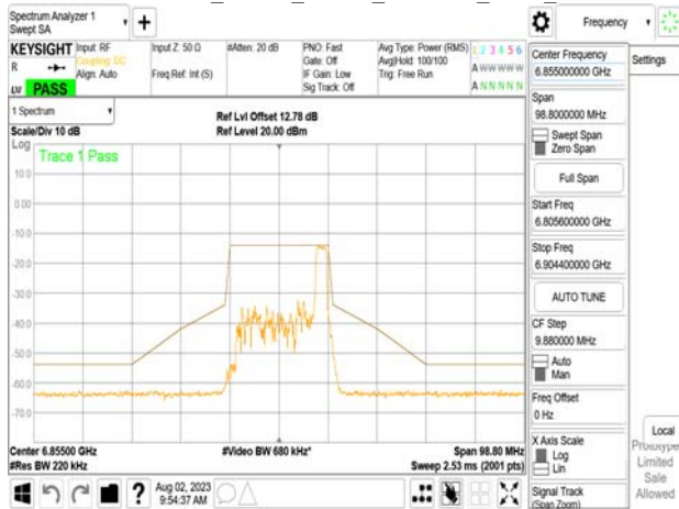
802.11ax_20MHz_Chain0_6855MHz_RU52_40
