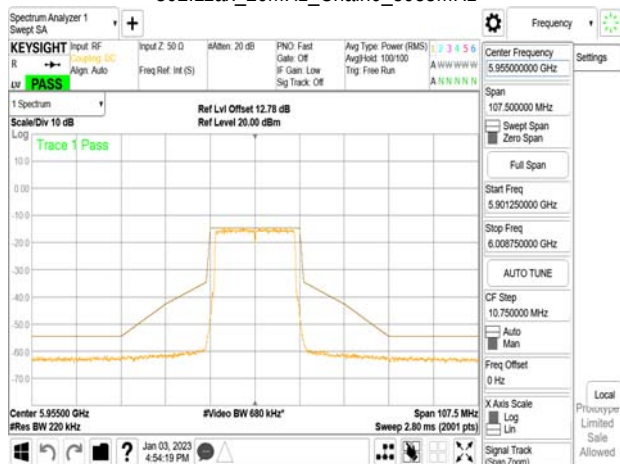
802.11ax_20MHz_Chain0_5955MHz_RU26_0
