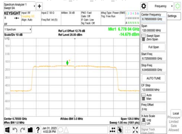
802.11ax_80MHz_Chain1_6785MHz_RU484_66
