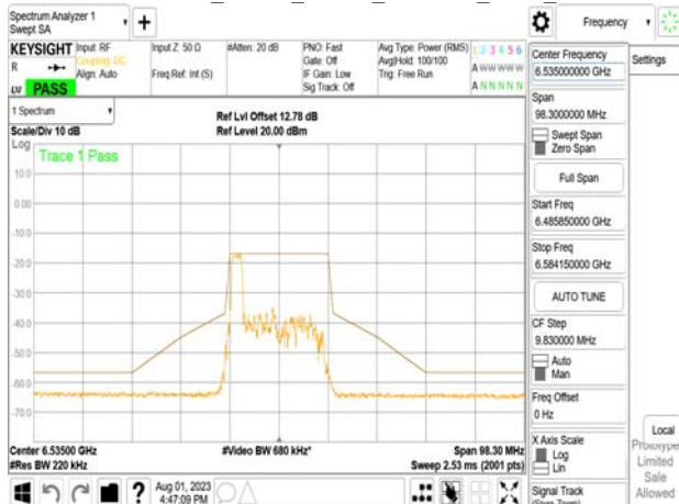
802.11ax_20MHz_Chain1_6535MHz_RU26_0
