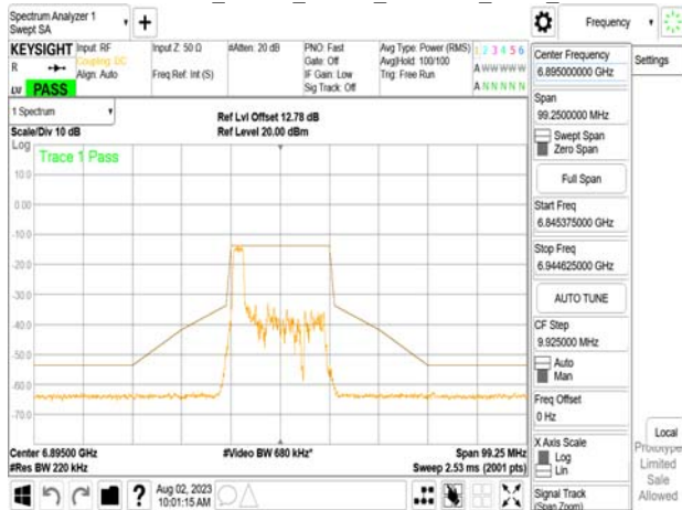
802.11ax_20MHz_Chain0_6895MHz_RU52_37
