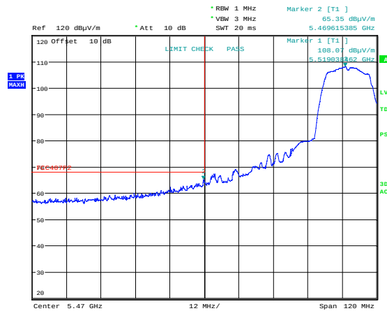
Band Edge 5470MHz, ch100, 802.11n SISO, Max
