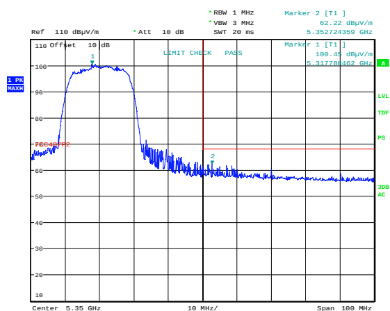
Band Edge 5350MHz, ch060, 802.11n MIMO, Max
