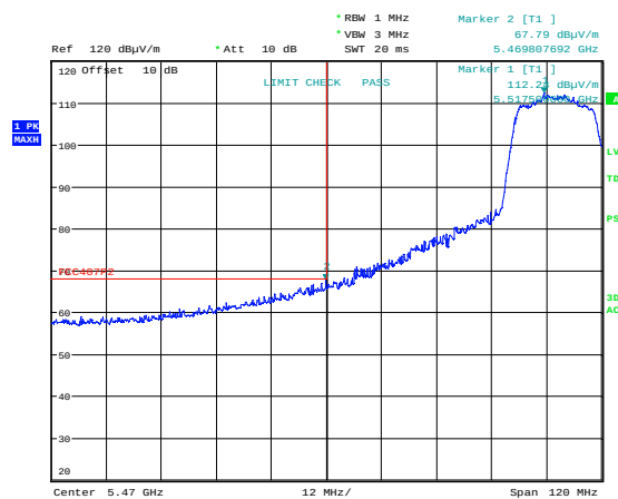
Band Edge 5470MHz, ch104, 802.11a 6M, Max
