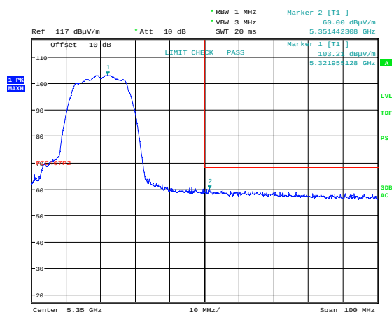
Band Edge 5350MHz, ch060, 802.11n SISO, Max
