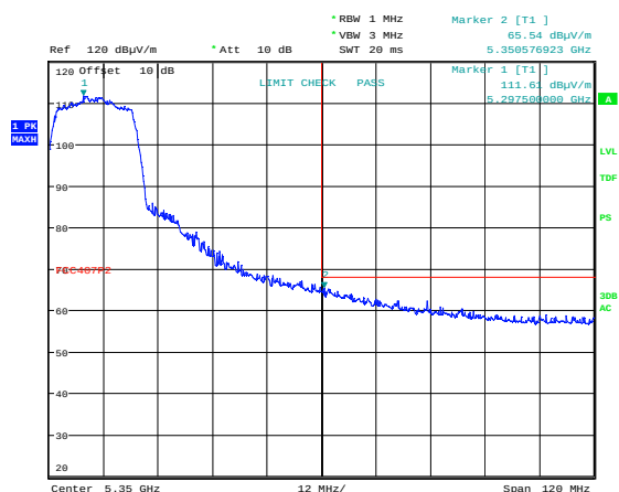
Band Edge 5350MHz, ch060, 802.11a 6M, Max
