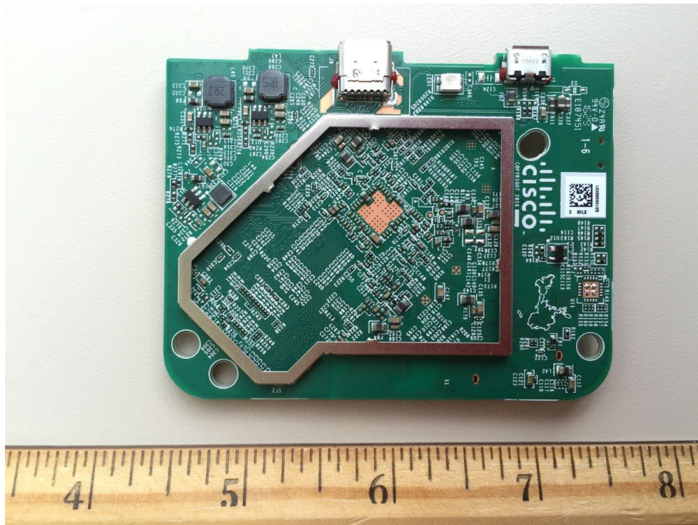
Top Side
