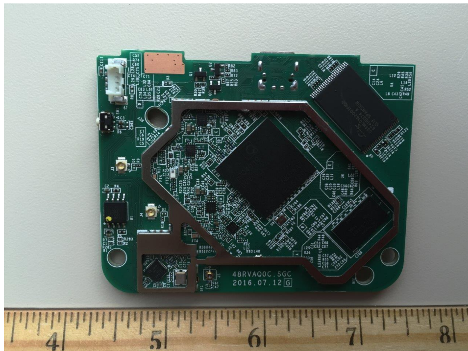
Bottom Side
