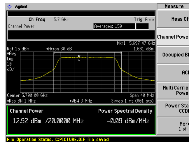
Ant-3
