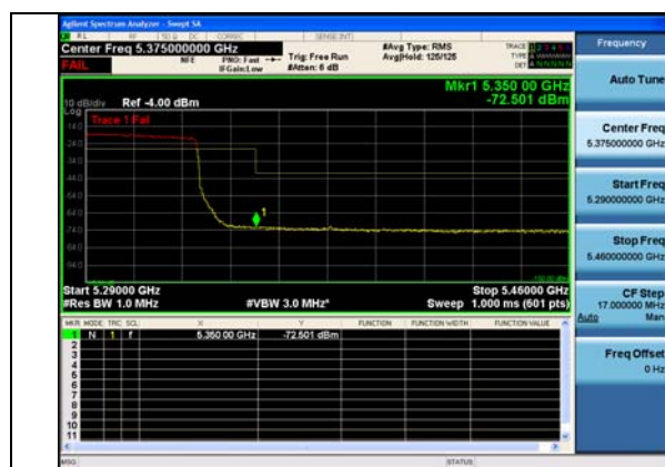
Antenna G
