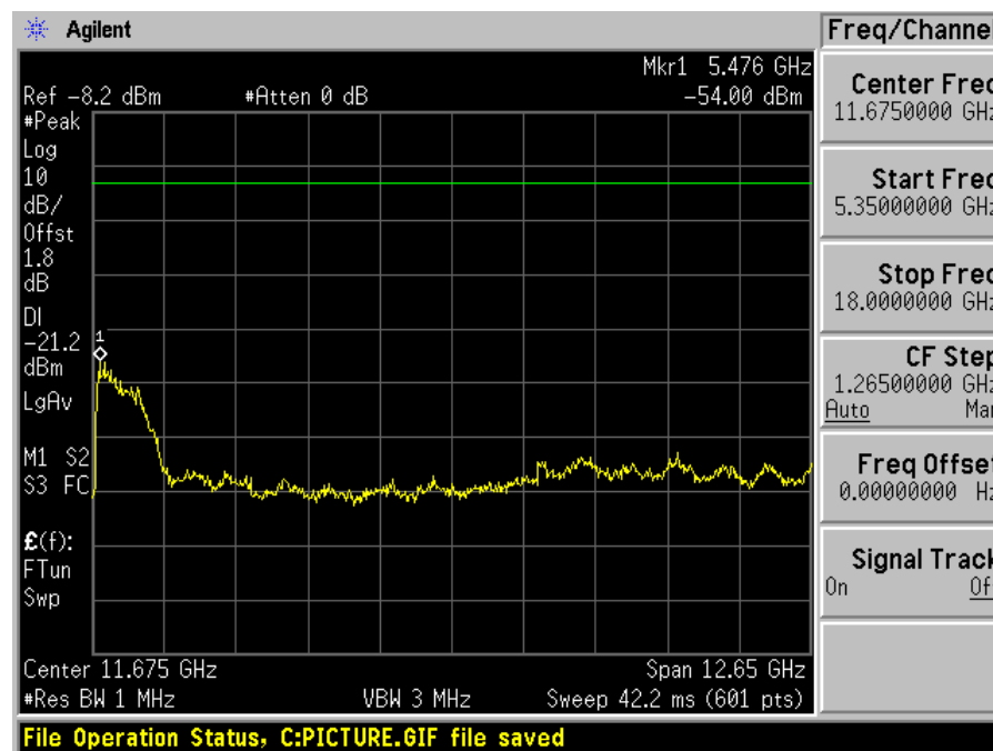
Ant-a-2
