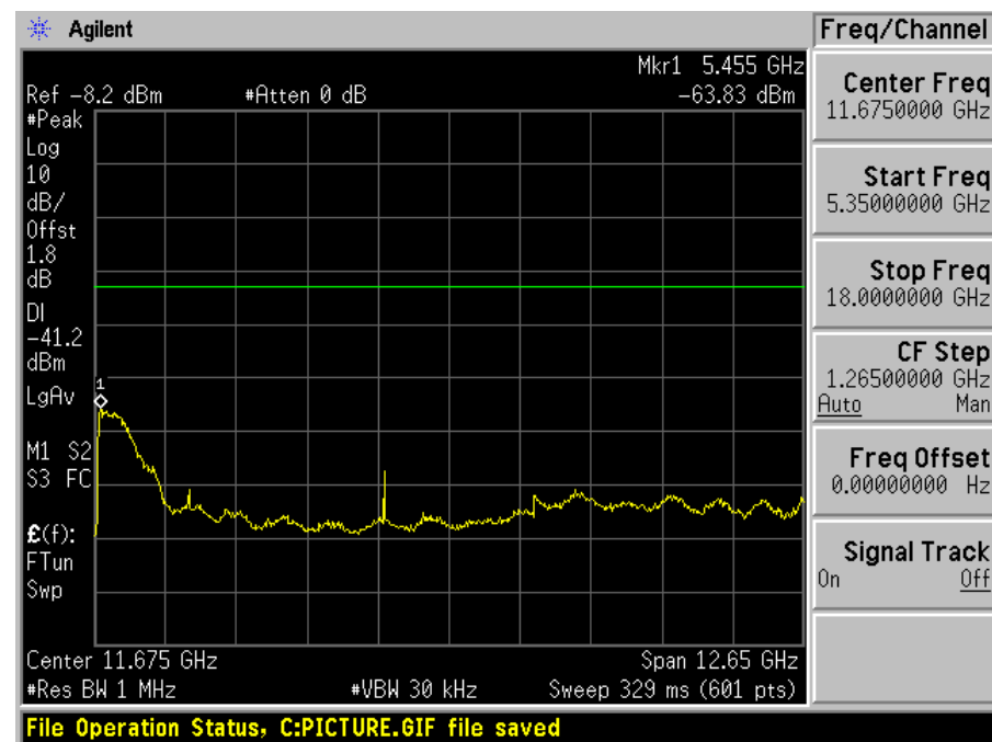
Ant-b-2
