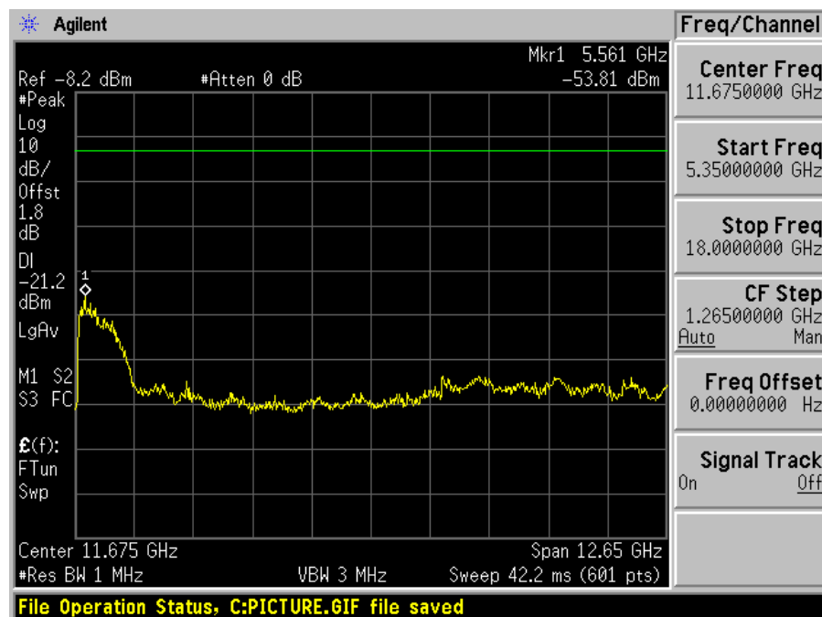
Ant-c-2
