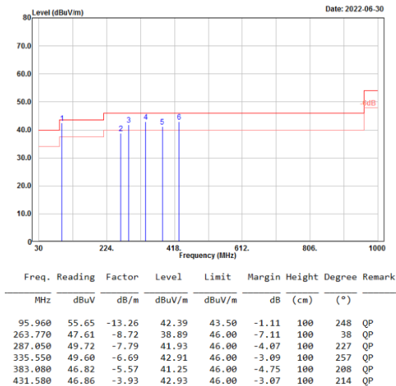
Mode 4 / Horizontal
