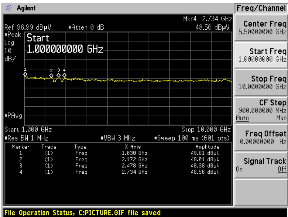
BLE 2480 1-10G-H-PK
