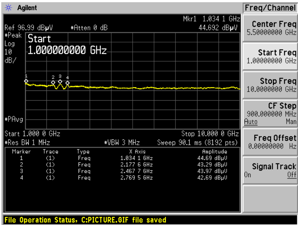
BLE 2480 1-10G-H-AV
