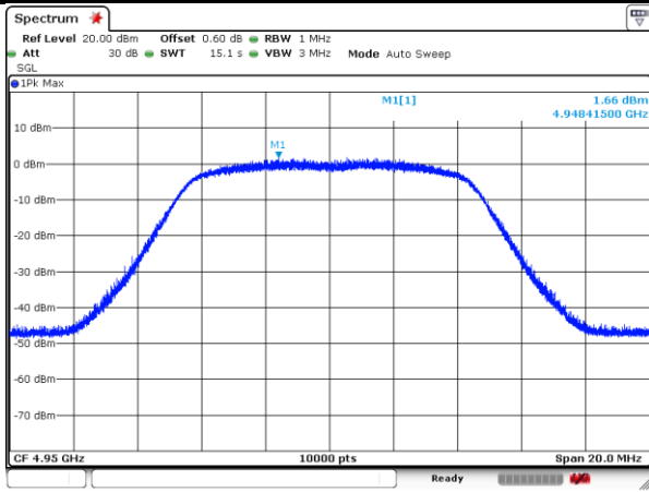
4950MHz-10MHz-802.11n-1-a
