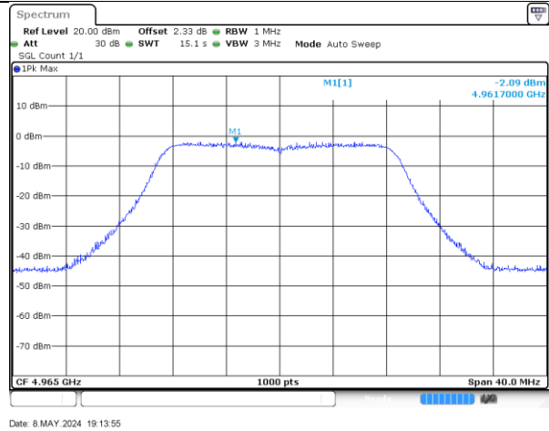
4965MHz-20MHz-802.11ac-2-b
