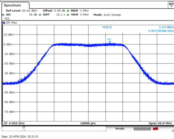
4955MHz-10MHz-802.11ac-1-a
