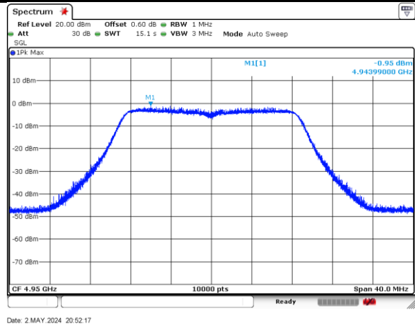
4950MHz-20MHz-802.11n-2-b
