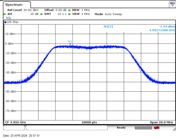
4955MHz-10MHz-802.11n-2-b
