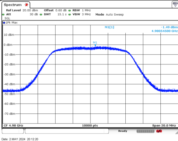
4980MHz-10MHz-802.11n-2-a
