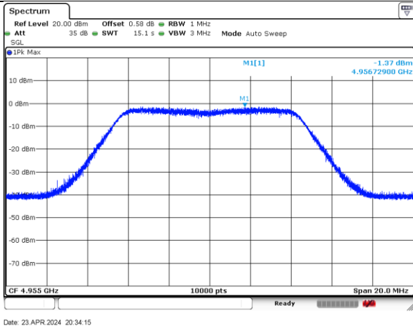
4955MHz-10MHz-802.11n-2-a
