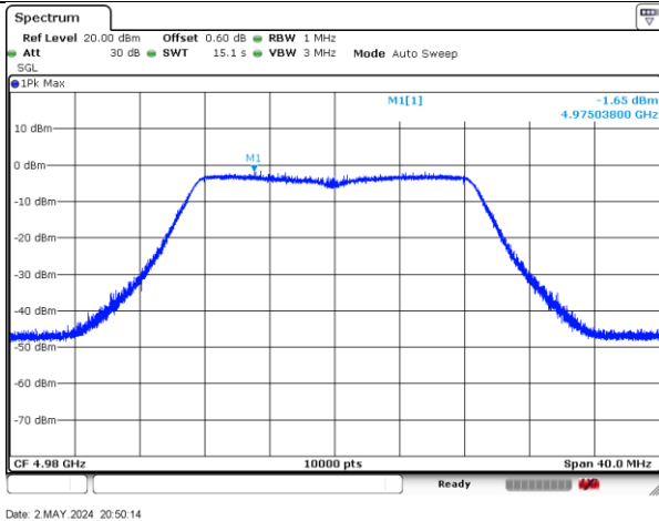
4980MHz-20MHz-802.11n-2-a
