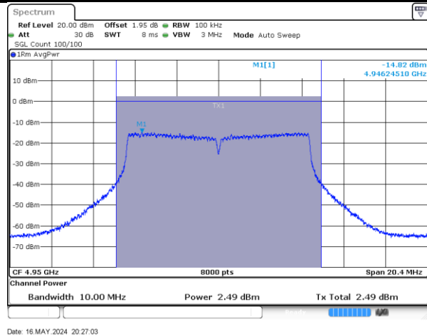
4950-10MHz-802.11ac-2-a
