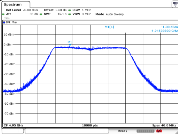
4950MHz-20MHz-802.11ac-2-a
