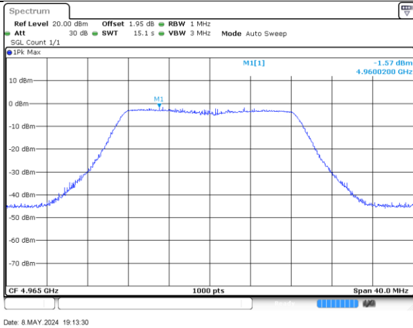
4965MHz-20MHz-802.11ac-2-a
