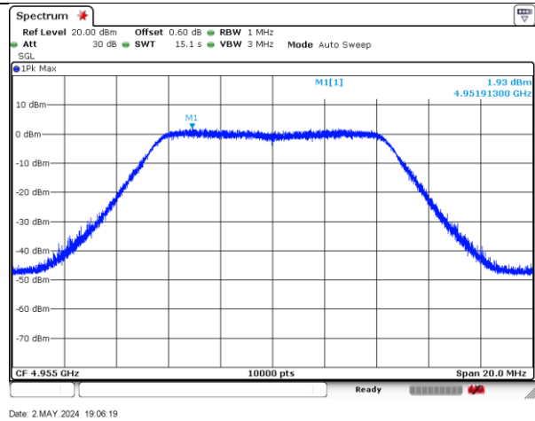
4955MHz-10MHz-802.11ac-1-b
