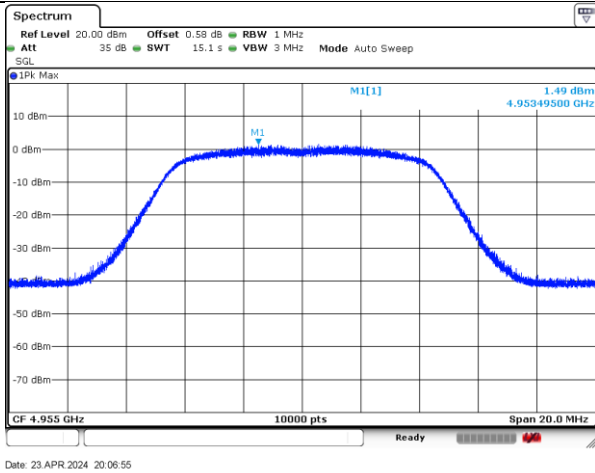
4955MHz-10MHz-802.11n-1-a
