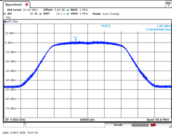
4955MHz-10MHz-802.11n-1-b
