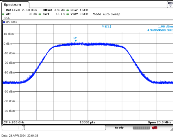
4955MHz-10MHz-802.11ac-1-a
