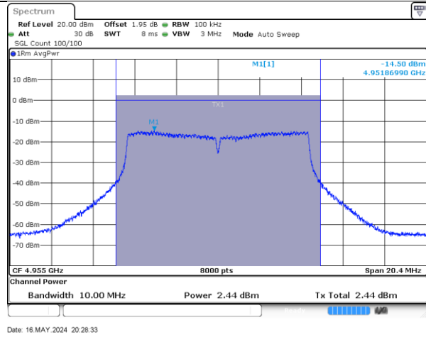
4955-10MHz-802.11ac-2-a
