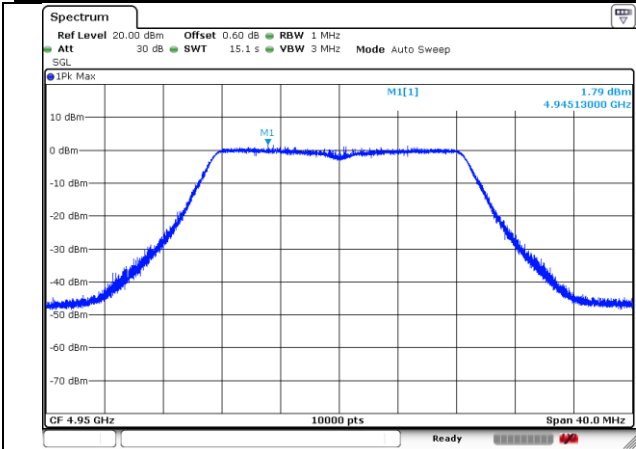
4950MHz-20MHz-802.11ac-1-a
