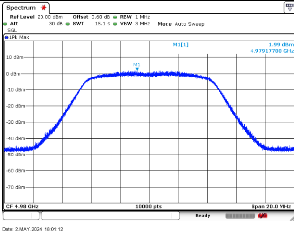
4980MHz-10MHz-802.11n-1-a
