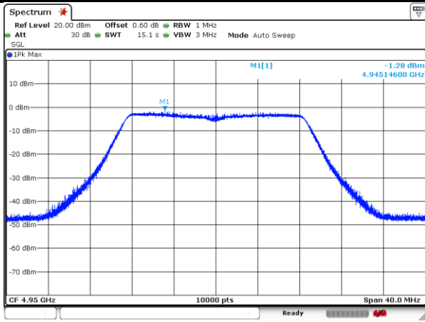
4950MHz-20MHz-802.11n-2-a
