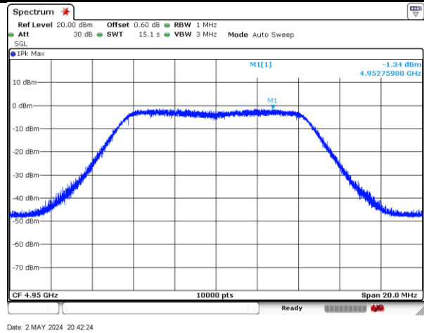
4950MHz-10MHz-802.11n-2-b
