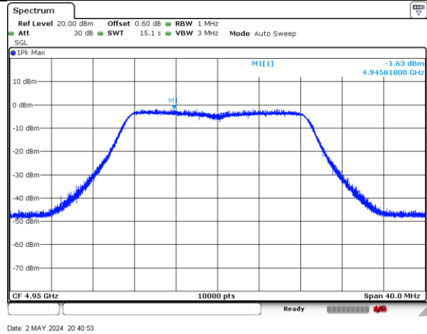
4950MHz-20MHz-802.11ac-2-b
