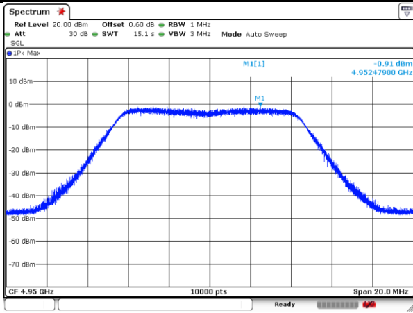
4950MHz-10MHz-802.11n-2-a
