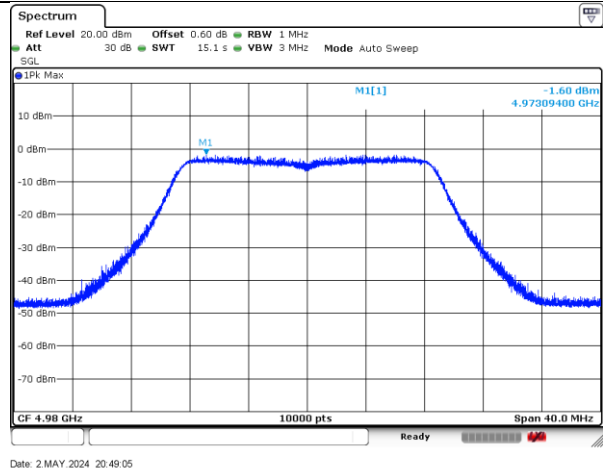
4980MHz-20MHz-802.11n-2-b
