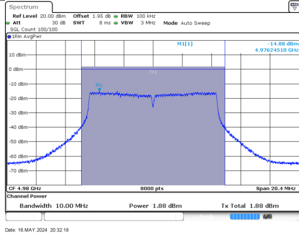
4980-10MHz-802.11ac-2-a
