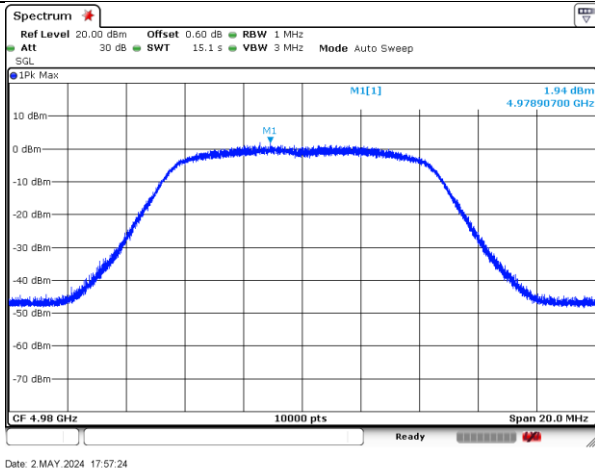
4980MHz-10MHz-802.11ac-1-a
