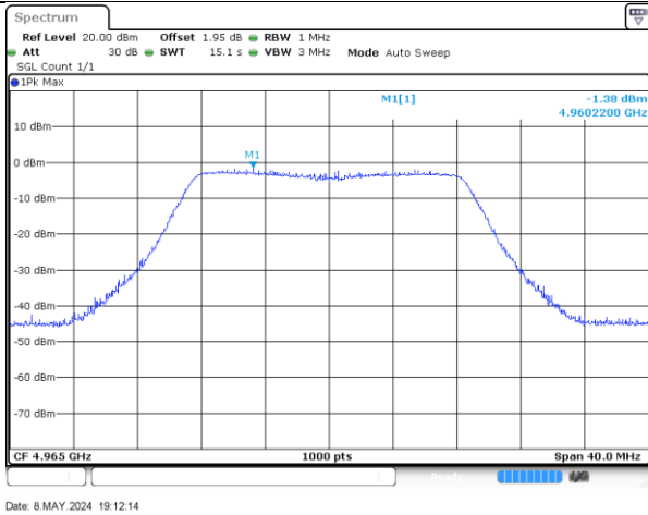
4965MHz-20MHz-802.11n-2-a
