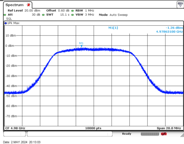
4980MHz-10MHz-802.11n-2-b
