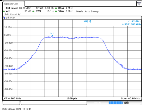
4965MHz-20MHz-802.11n-2-b
