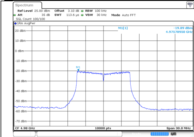
4980-10MHz-802.11ac-2-a
