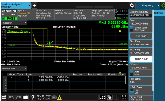
Antenna A
