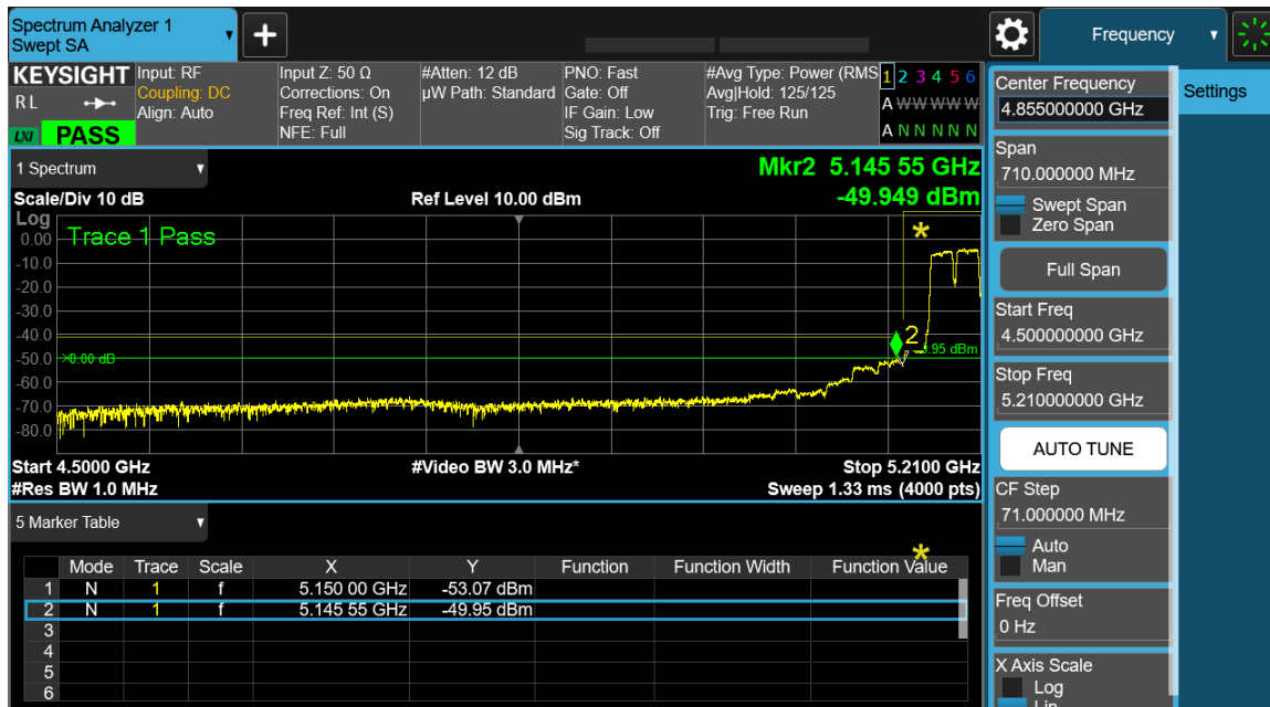
Antenna A
