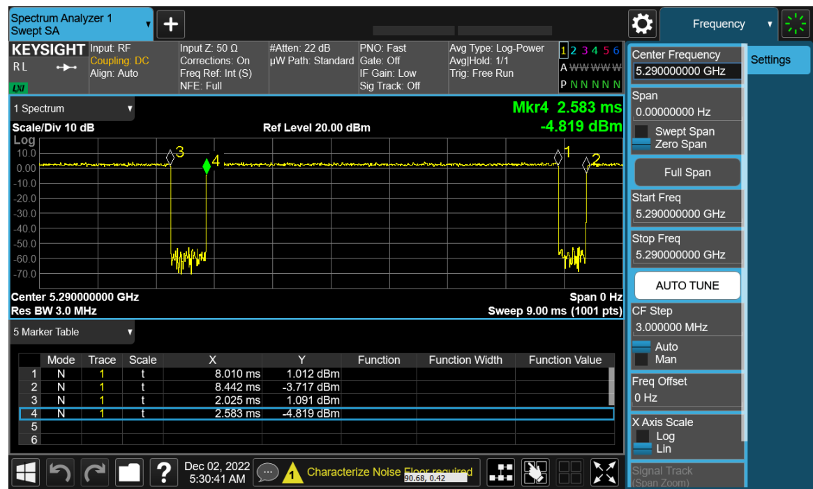
Antenna A
