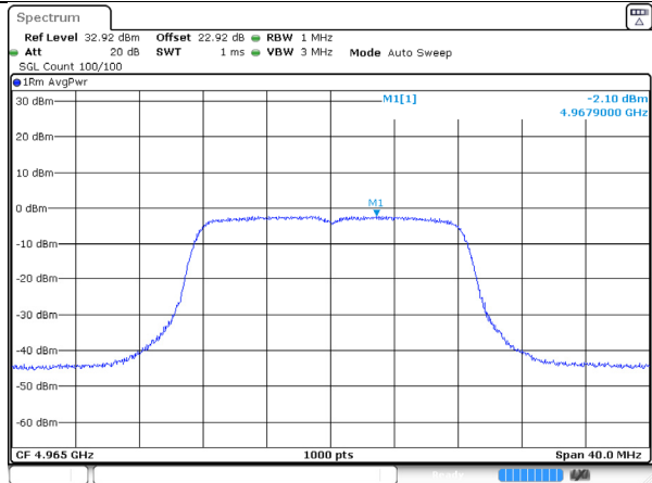
4965MHz-tx1-cobalt_13
