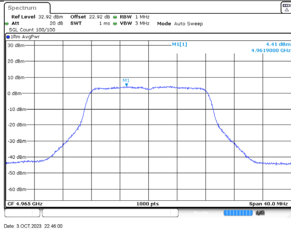
4965MHz-tx2-cobalt_16
