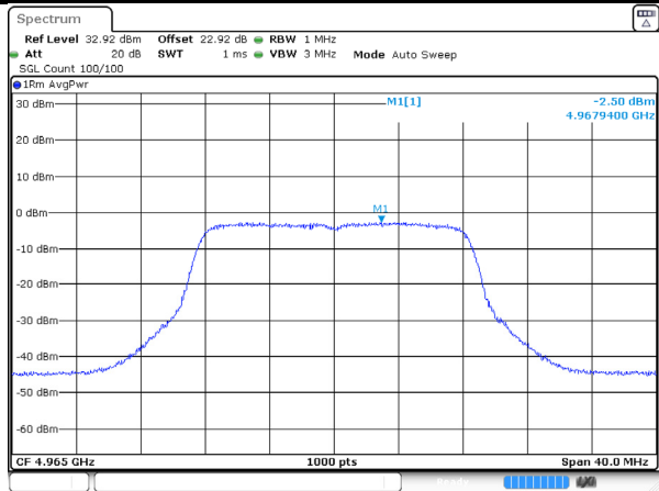
4965MHz-tx1-cobalt_13
