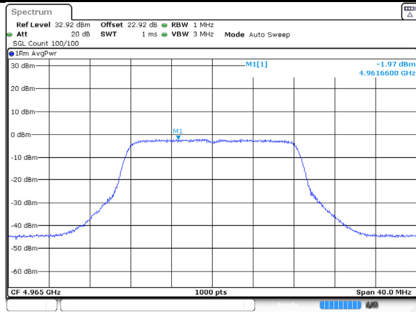
4965MHz-tx2-cobalt_11
