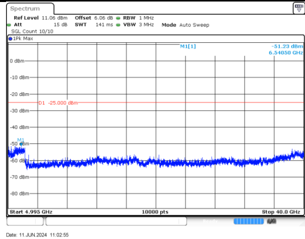
4955-10MHz-802.11a-2-b
