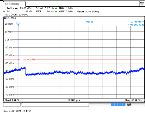
4980-10MHz-802.11a-1-a
