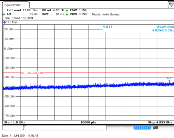
4955-10MHz-802.11a-2-b
