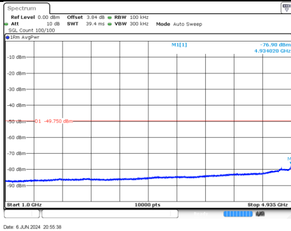
4965-20MHz-802.11n-2-b
