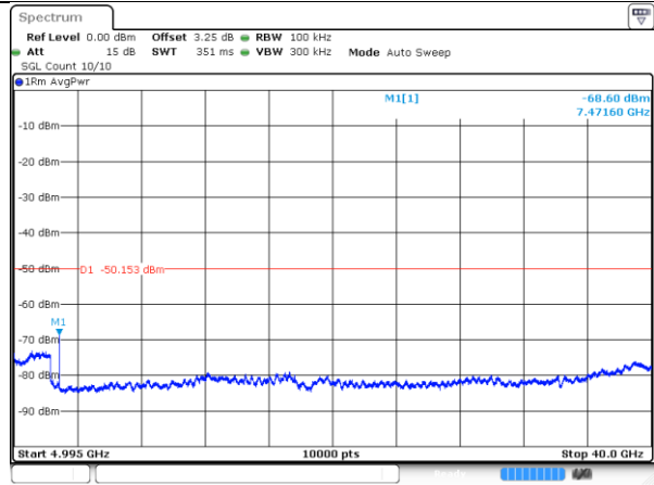
4980-10MHz-802.11ac-1-a
