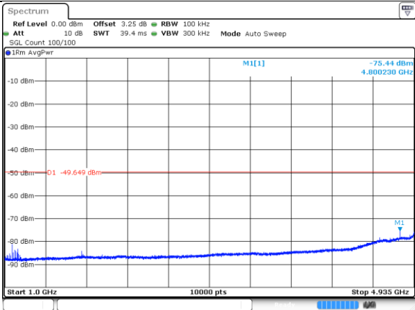
4965-20MHz-802.11n-2-a
