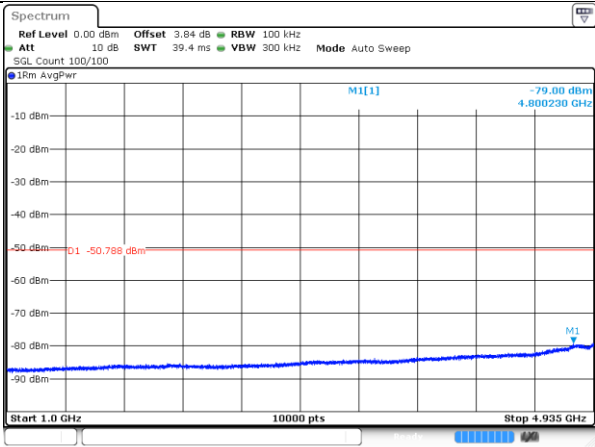
4980-20MHz-802.11n-2-b
