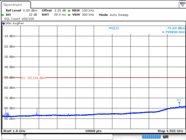
4980-20MHz-802.11n-2-a
